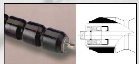
Selbstreinigende Rücklaufrollen
